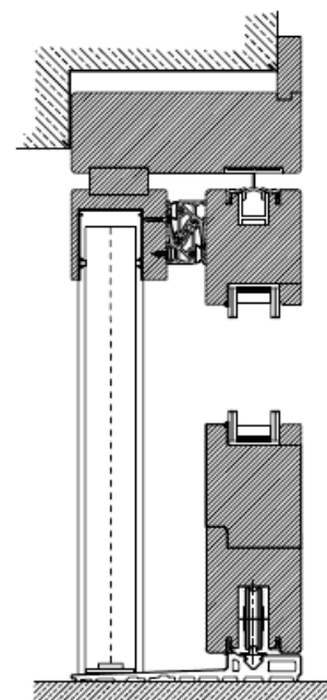
Sezione verticale vertical section
