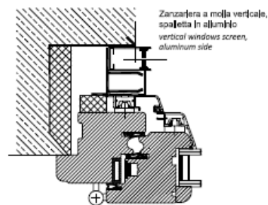
Sezione orizzontale horizontal section
