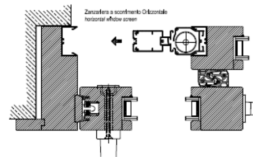
Sezione orizzontale horizontal section
