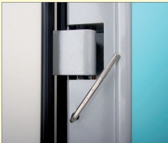
CERNIERA A SCOMPARSA registrazione verticale.
